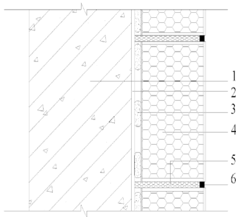
图 6.7.1 保温装饰板系统
