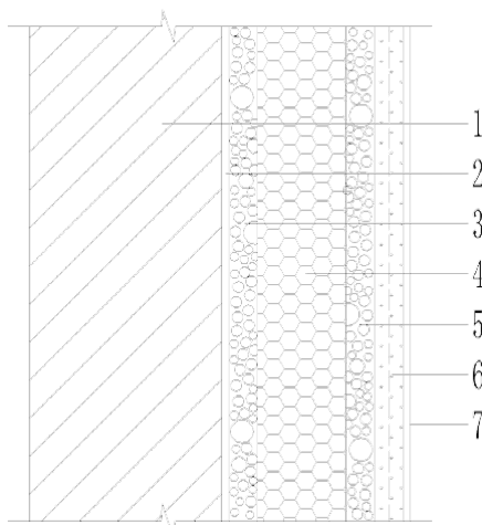
图 6.5.1 保温板贴砌系统
