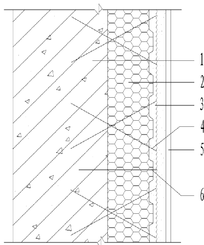
图 6.4.1 有网现浇系统
