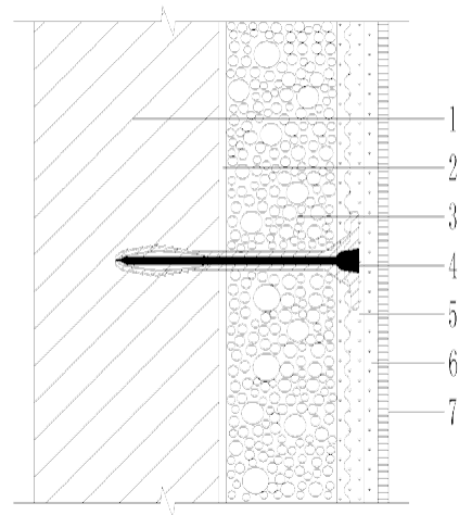
图 6.2.1-2 面砖饰面保温浆料系统
