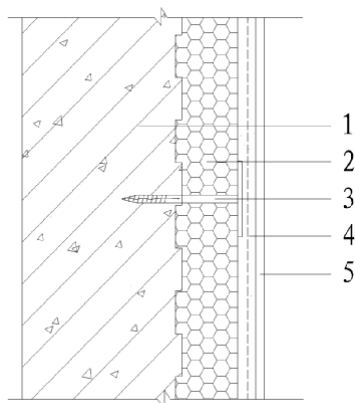
图 6.3.1 无网现浇系统
