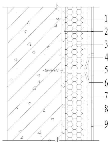
6.1.2 EPS 板面砖饰面系统
