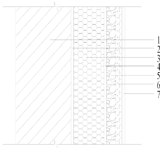
图 6.6.1 PU 喷涂系统
