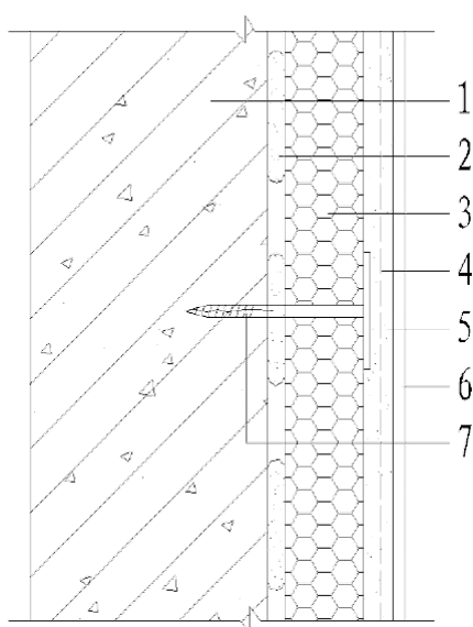
图 6.1.1 粘贴保温板涂料饰面系统图
