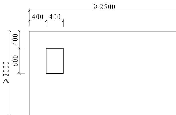
图 A.2.1 基层墙体
