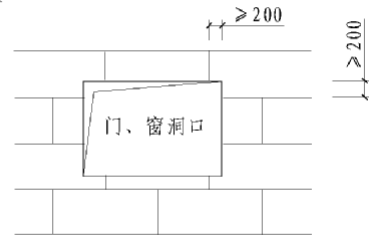
图 6.1.9-2 门窗洞口保温板排列
