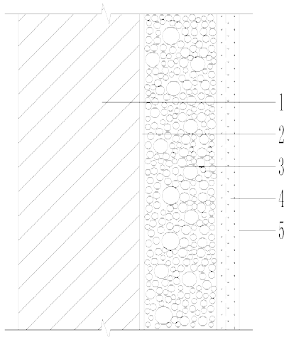
图 6.2.1-1 涂料饰面保温浆料系统
