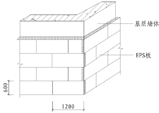
图 6.1.9-1 保温板排版图
