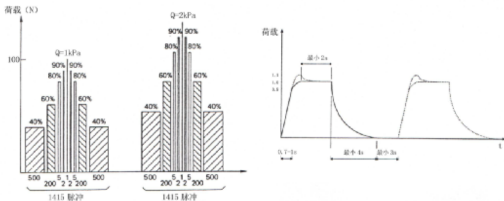
图 A.3.3 加压步骤及压力脉冲图形
