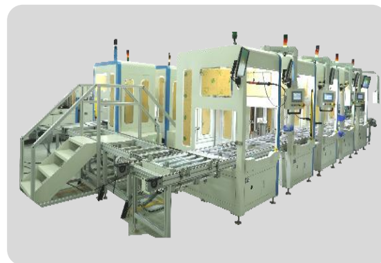
新能源发动机自动装配线 NEV Motor Assembling Line
